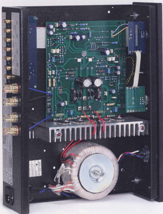
Der Ringkerntrafo ist durch den Kühlkörper abgeschirmt, der Signalweg von der Vorverstärkerplatine bis zu den Lautsprecherklemmen ist nicht länger als nötig
